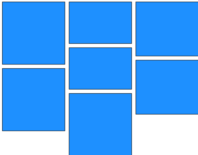
Tile List
